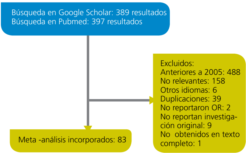
Figura A. 3: Flujograma de resultados de la búsqueda sistemática de MA
