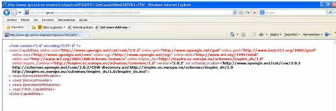
Figura 10.3.- Secciones principales de la respuesta a la petición GetCapabilities
