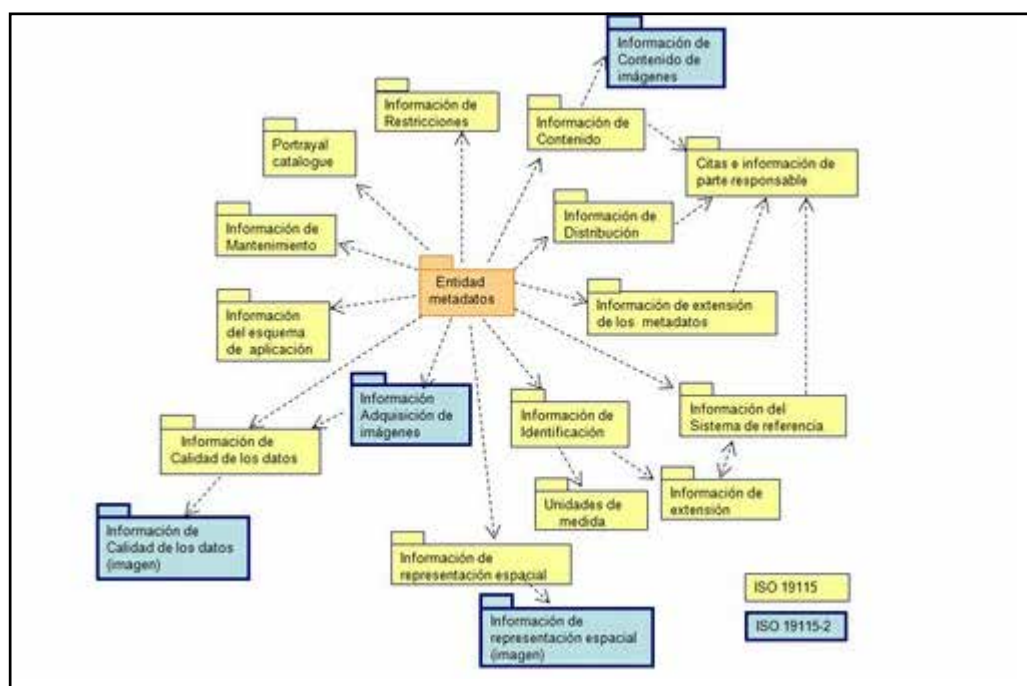
Figura 13.3. -Paquetes de metadatos de la Norma ISO 19115-2 y su relación con la Norma ISO 19115 (fuente: revista Mapping, N° 123)
