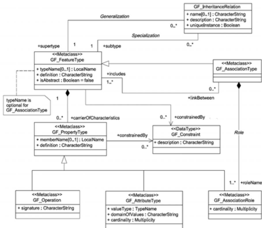
Figura 3.27.- Fragmento de GFM
