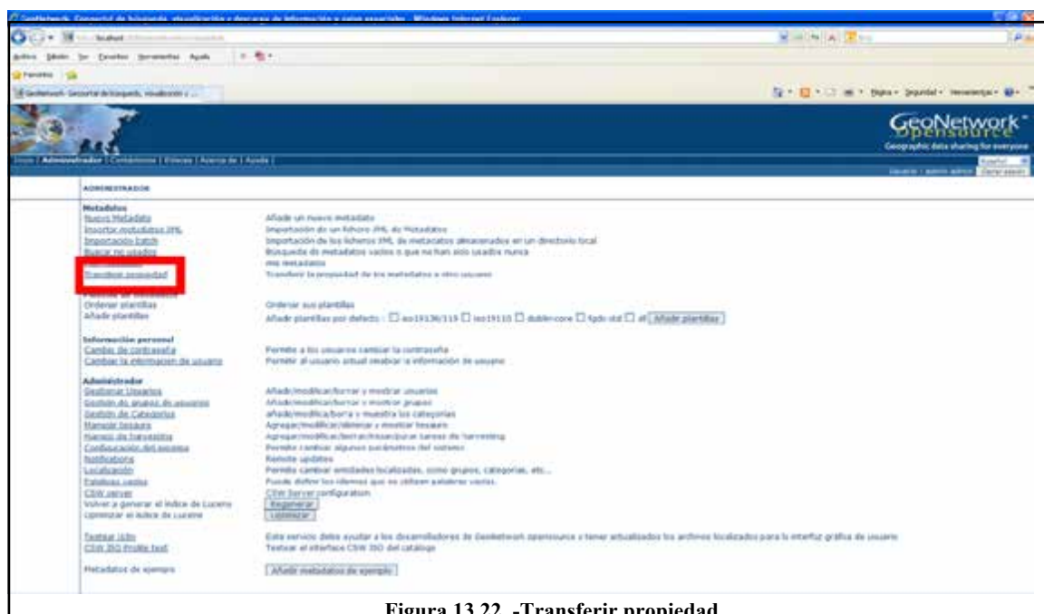
Figura 13.22. -Transferir propiedad
