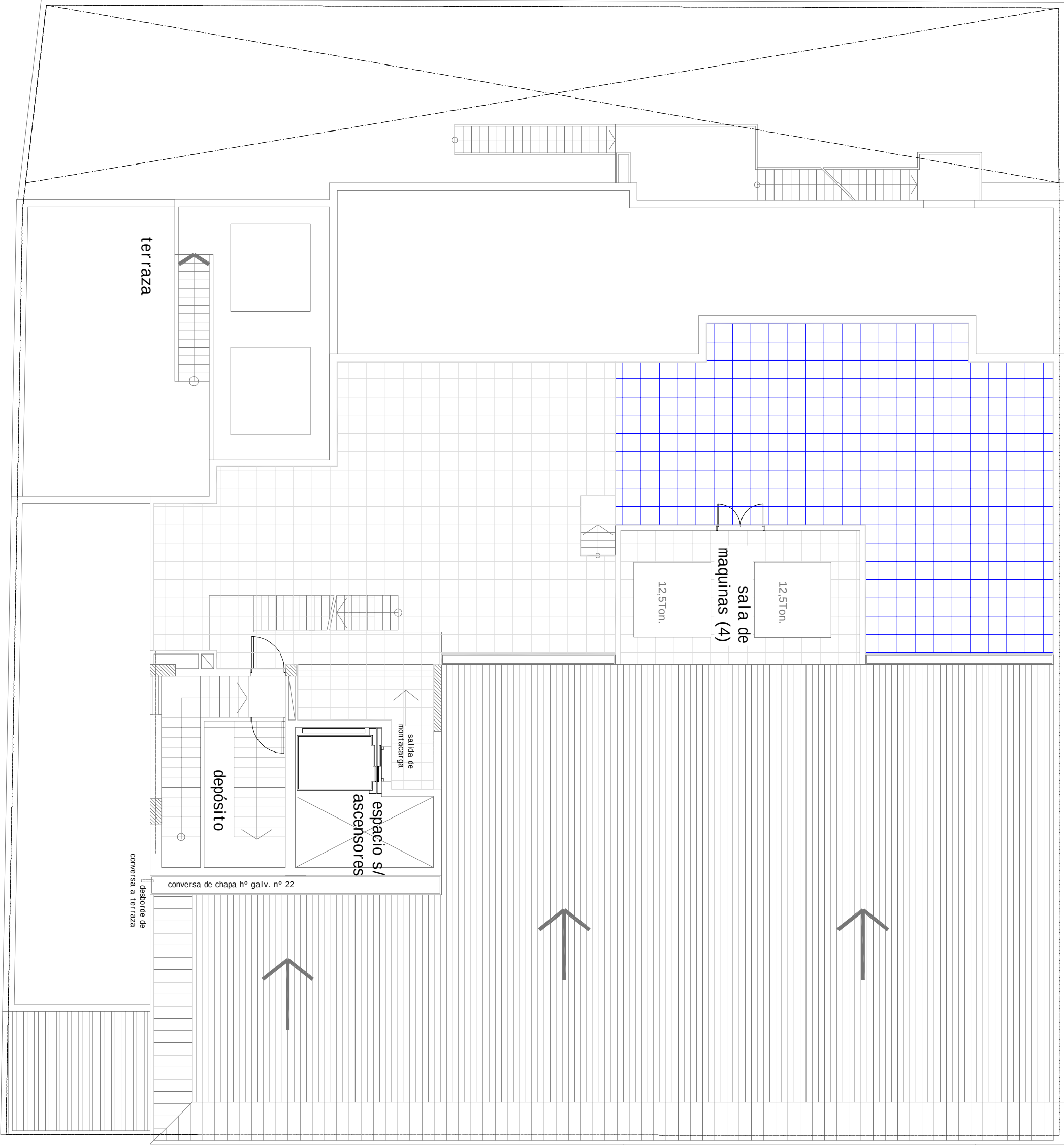
PLANTA TERRAZA
