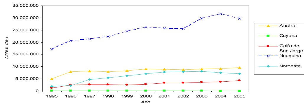
Gráfico 7: Evolución de la producción de gas natural por cuenca. Total del país. Años 1995-2005
