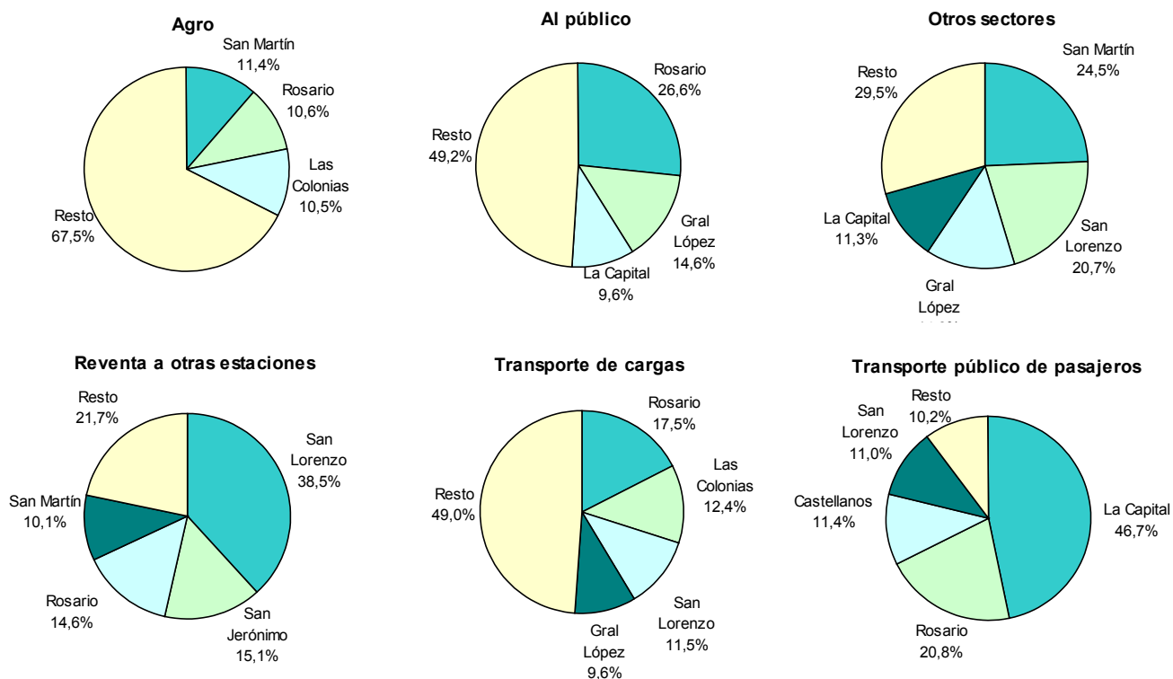
Gráfico 15: Participación de los departamentos en el volumen de venta de combustibles por canal de comercialización. Provincia de Santa Fe. Año 2005
