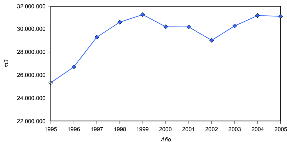
Gráfico 12: Evolución del volumen de petróleo procesado. Total del país. Años 1995-2005
